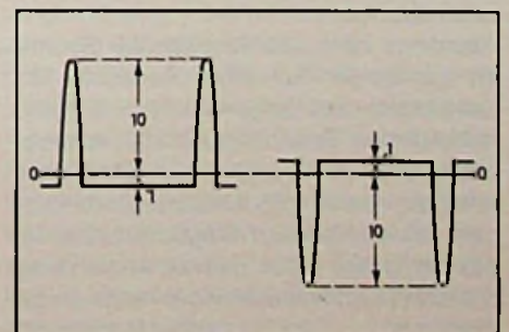
Bild 3. Die Thyristoren der SSVD-Schaltung müssen den hohen Zeilenrückschlag-Impulsen standhalten. Der Wert der Zeilenhinlauf-Spannung ist um den Faktor 10 niedriger
