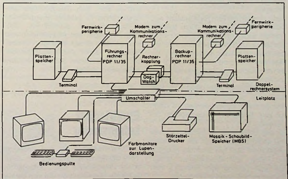
Bild 3. Leitstelle mit Doppelrechnersystem und Leitplatz, die räumlich getrennt sind
