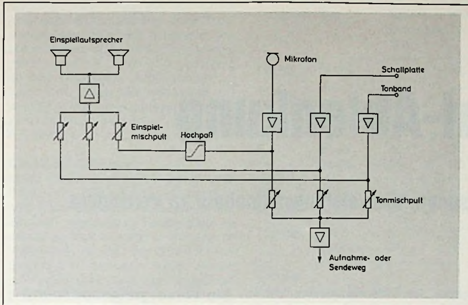
Bild 2. Grundschieltung einer Einspielanlage. Mikrofon-, Schallplatten- oder Tonband-Darbietungen werden von den Einspiellautsprechern wiedergegeben. Der Hochpaß im Mikrofonzweig senkt die Gefahr einer akustischen Rückkopplung. Über das Tonmischpult kann die Einspielung aufgezeichnet oder live gesendet werden.
