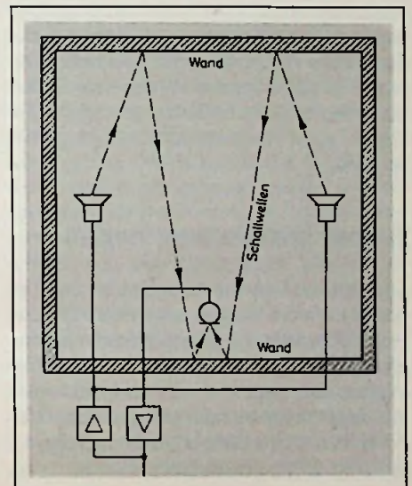
Bild 1. Die Lautsprecher und das Mikrofon sind hier richtig aufgestellt, denn sie kehren sich gegenseitig „den Rücken“ zu. Dennoch kann es über indirekte Schallwege aufgrund von Reflexionen zur akustischen Rückkopplung kommen.
